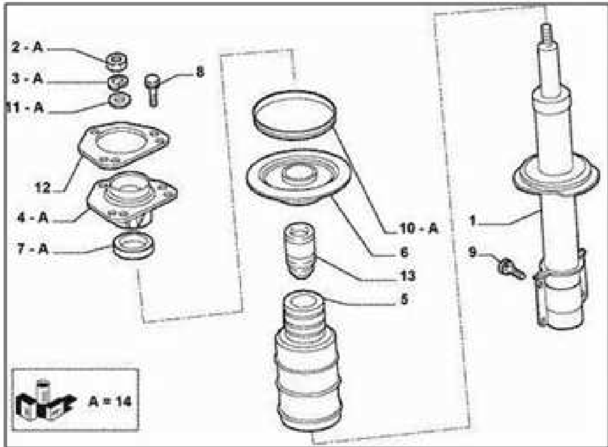
Складальне креслення
