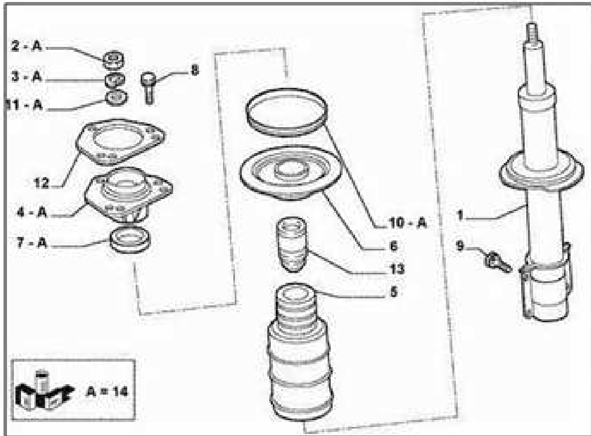
Складальне креслення
