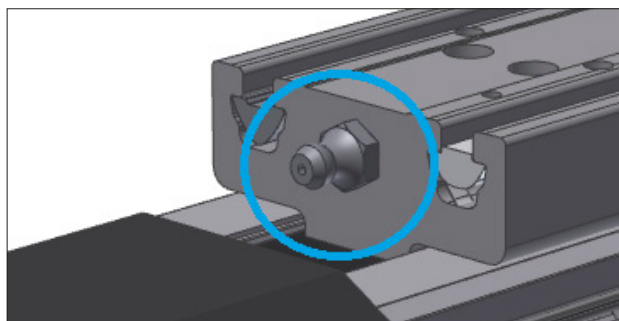
Bild 4.3 Schmierstellen bei AXE60Z, AXE80Z, AXE100Z
