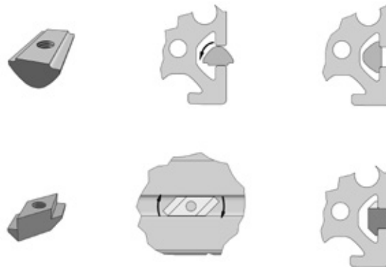
Bild 6.3 Bauformen von Nutensteinen
