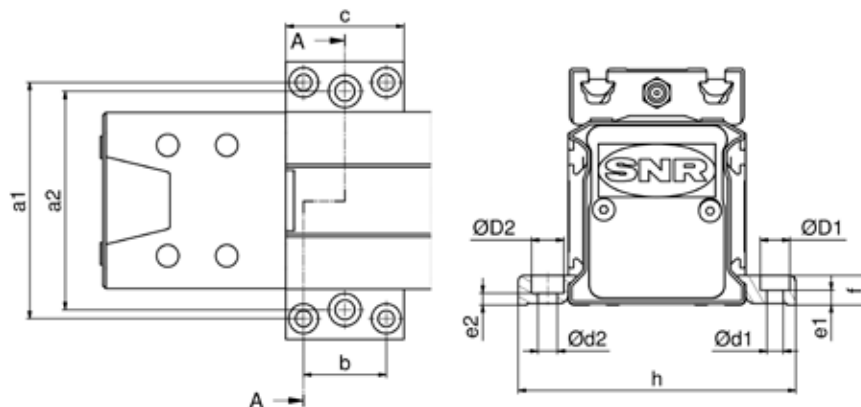
Bild 6.2 Abmessungen Befestigungsleisten AXE
