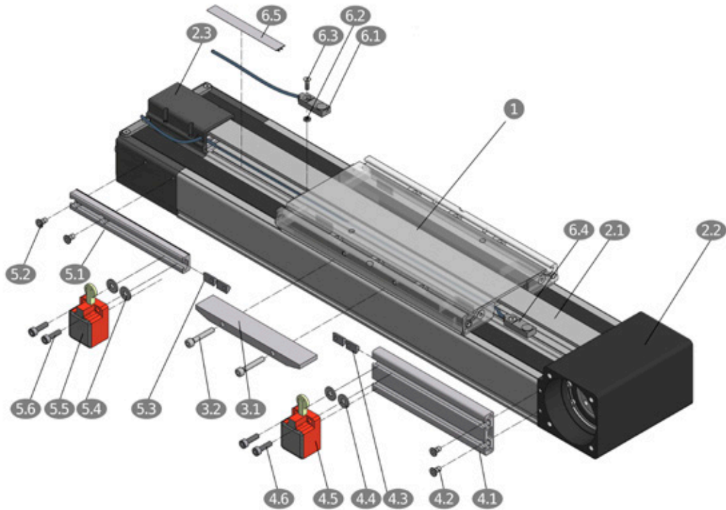
Bild 3.14 Montage von Endschaltern an Linearachsen AXE110Z
