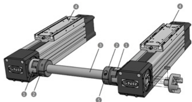
Bild 3.11 Montage von Parallelen Linearachsen mit Verbindungswelle
