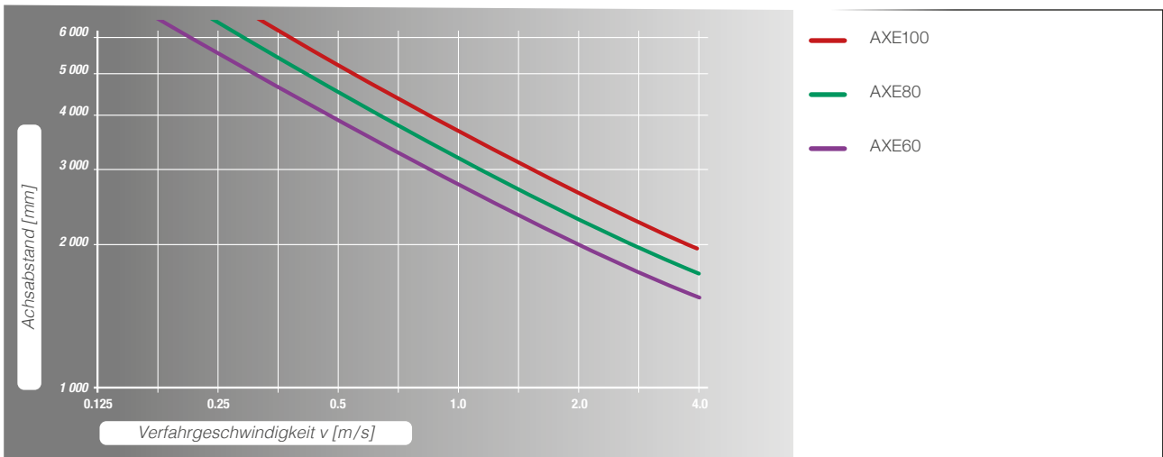
Bild 6.27 Dynamische Grenzwerte von Verbindungswellen
