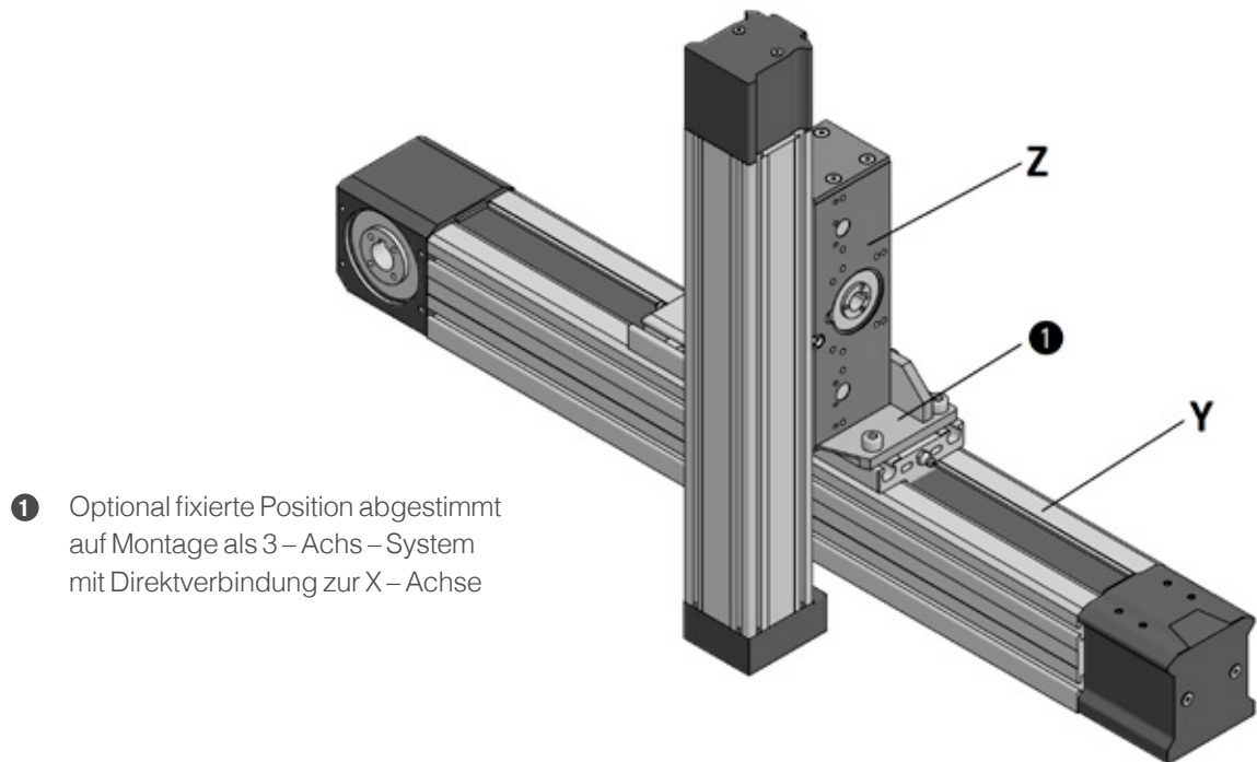
Bild 6.10 A - Standardverbindung AXE
