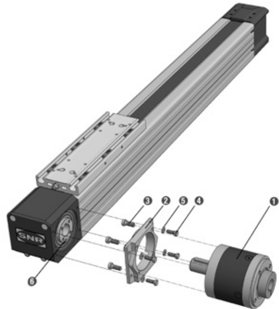
Bild 3.5 Formschlüssige Getriebemontage an Linearachsen mit Zahnriemenantrieb
