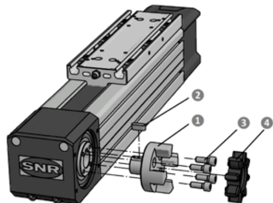
Bild 3.6 Kraftschlüssige Kupplungsmontage an Linearachsen mit Zahnriemenantrieb
