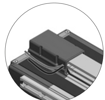
Bild 3.15 Leitungsführung für induktive Näherungsschalter AXE110Z
