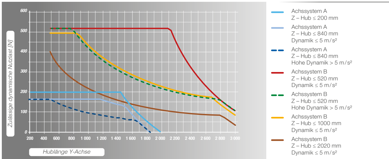
Bild 7.2 Dynamische Nutzlast von Standard - Achssystemen
