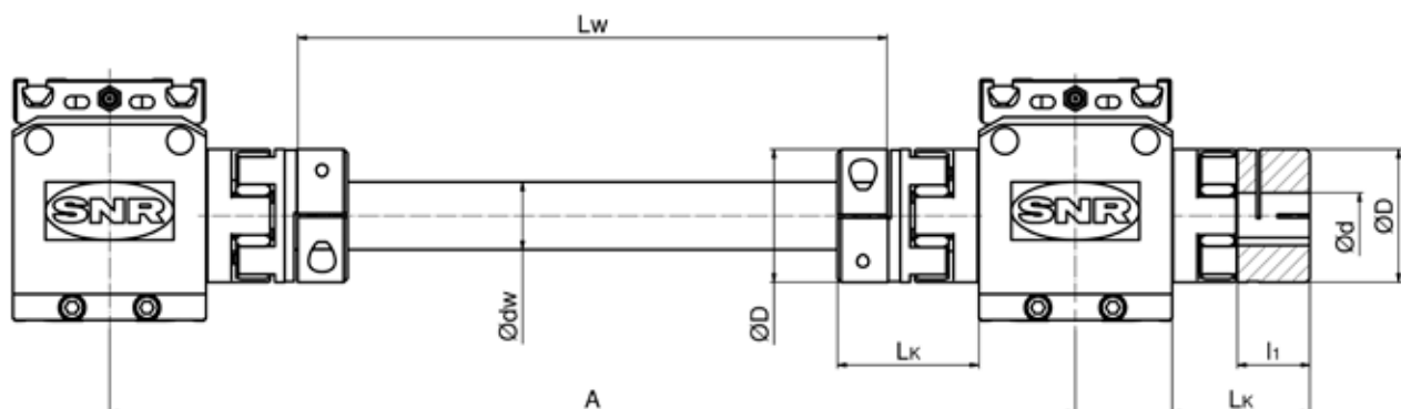
Bild 6.19 Abmessungen Kupplungen und Verbindungswelle
