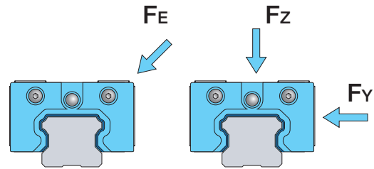
Bild 2.2 — Äquivalente Belastung
