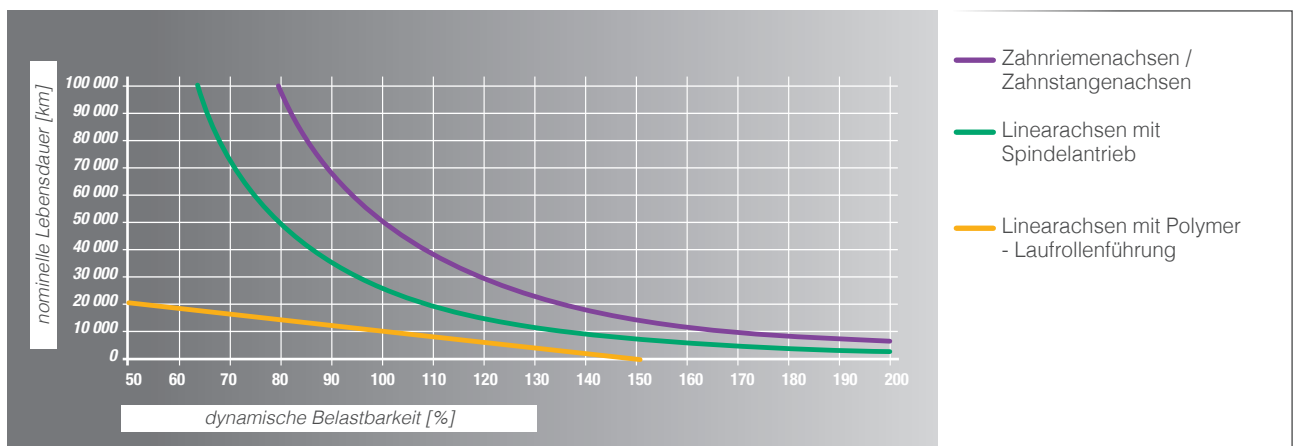
Bild 2.3 — Nominelle Lebensdauer
