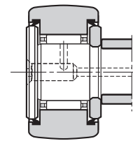
KR -- LL (mit Käfig, abgedichtet)
