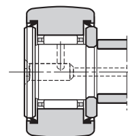
KR -- LL (mit Käfig, abgedichtet)
