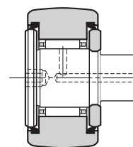
KR -- LLH (mit Käfig, abgedichtet)
