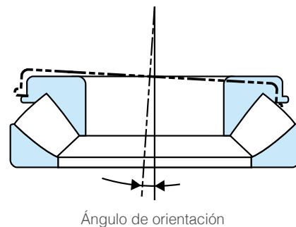
Desalineaciones admisibles
