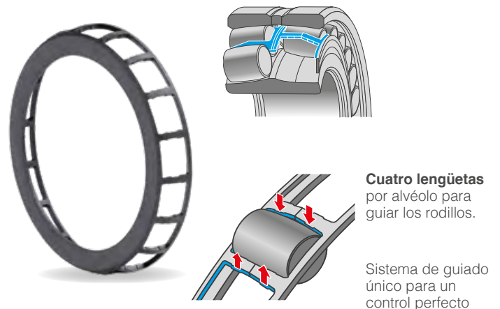
EA – Jaula de chapa de acero
