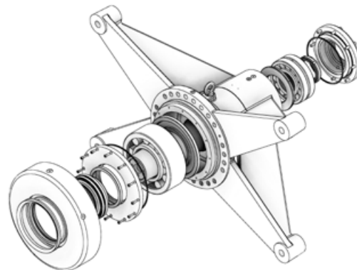
Ejemplo: módulo personalizado listo para instalar en una lavadora industrial
