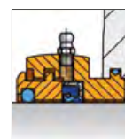
Junta de taconite Sello múltiple para entornos difíciles
