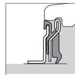
Étanchéité L4
