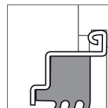
Étanchéité L3
