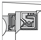
Étanchéité I
