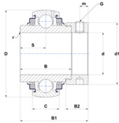
Type EX
