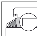
Уплотнение B
