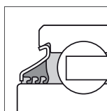
Уплотнение В
