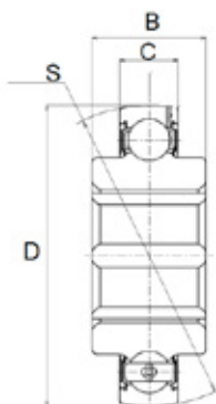
Тип 2
